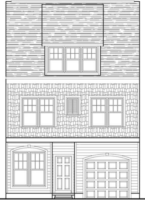
Elevation "C"
